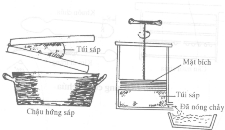
Hình 20. Bộ ép sáp đơn giản
